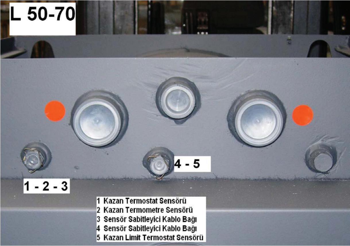
L 50 – L 70 sensör montajı
