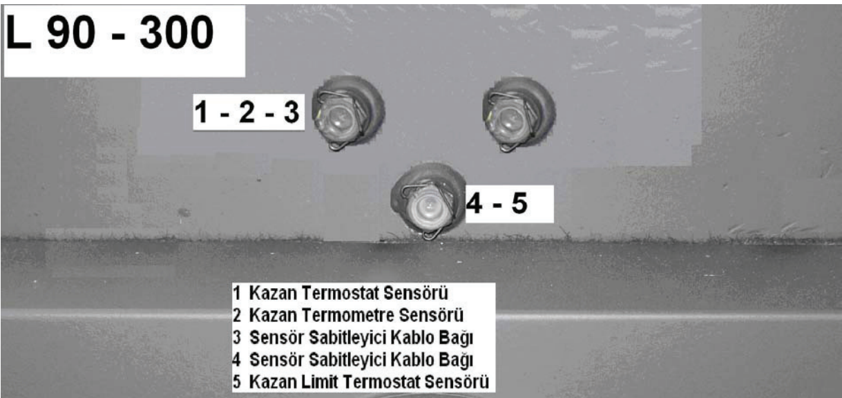
L 90 – L 300 sensör montajı
